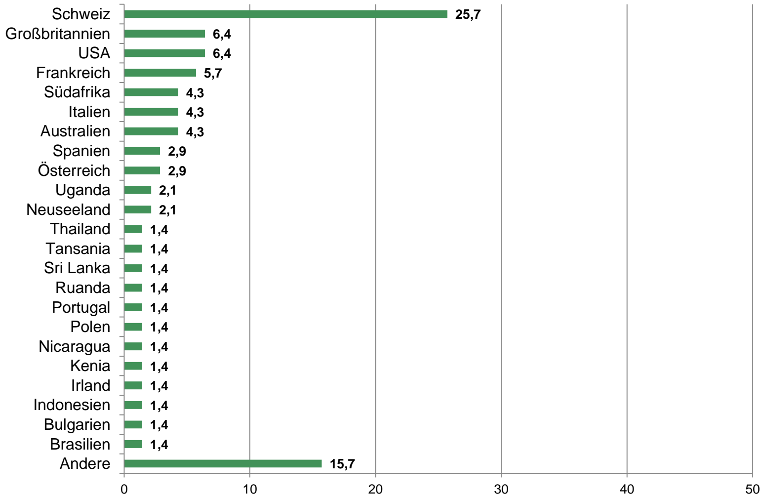
Auslandsaufenthalte: Länder (%)
